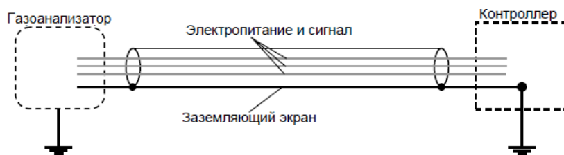
Рисунок 13 – Заземление экранированного кабеля
