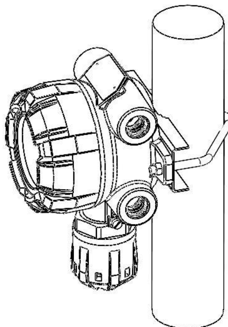
Рису- – Вид лиза- тора, уста- нов- ного лен- на трубу
