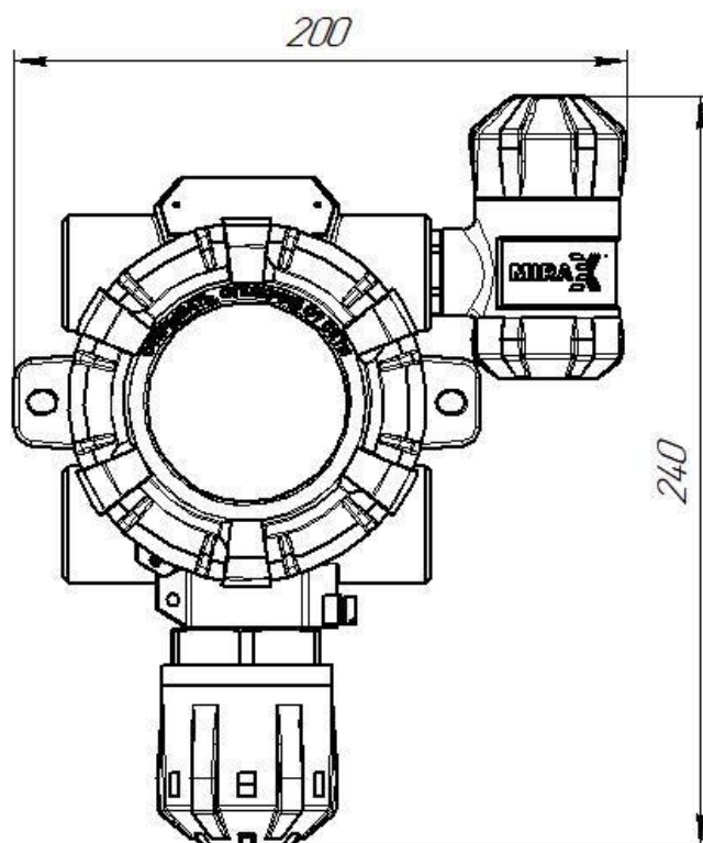
Рисунок 2 – Габаритные размеры AXIOM
