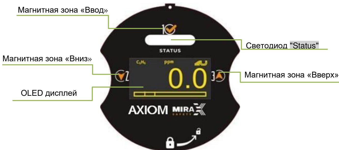
Рисунок 4– Лицевая панель AXIOM
